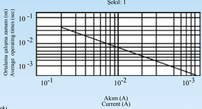
Şekil 1: Parafudr Ayırıcıları Akım-Ortalama Çalışma Zamanı Eğrisi.
