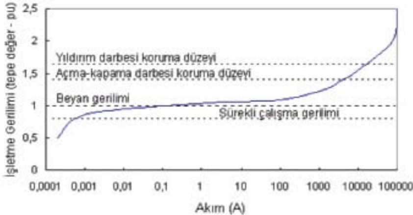
Metal oksit parafudrda akım- gerilim karakteristiği (sembolik)
